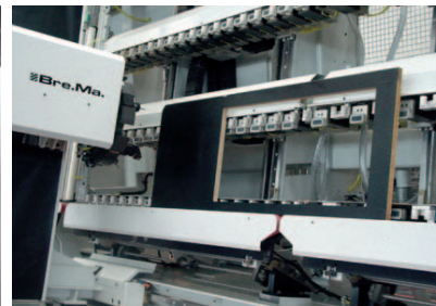
Centro Verticale di Foratura - Fresatura
