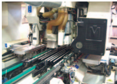
Centro di Foratura - Fresatura
